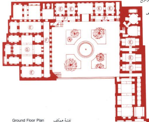
Ground Floor Plan نقشه همکف
